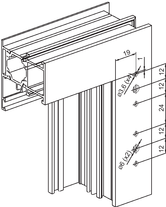
Otworky pod wspornik zawiasy górnej TwO 6 Szablon Nr 1AW0210XX
